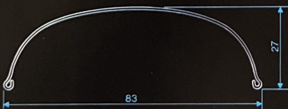
profilo anteriore mod. S 9500 G
