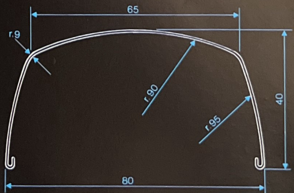
profilo posteriore mod. S 9380
